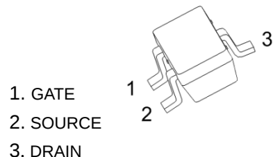
SOT-23-3L
